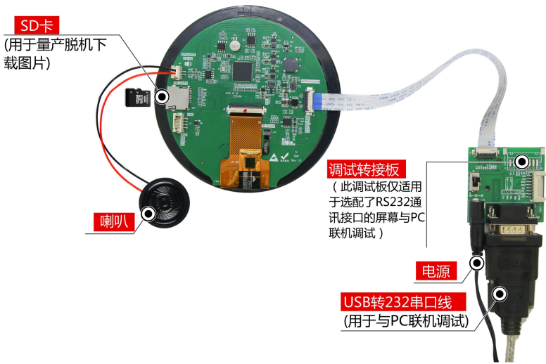
图 1-3RS232 调试工具图
